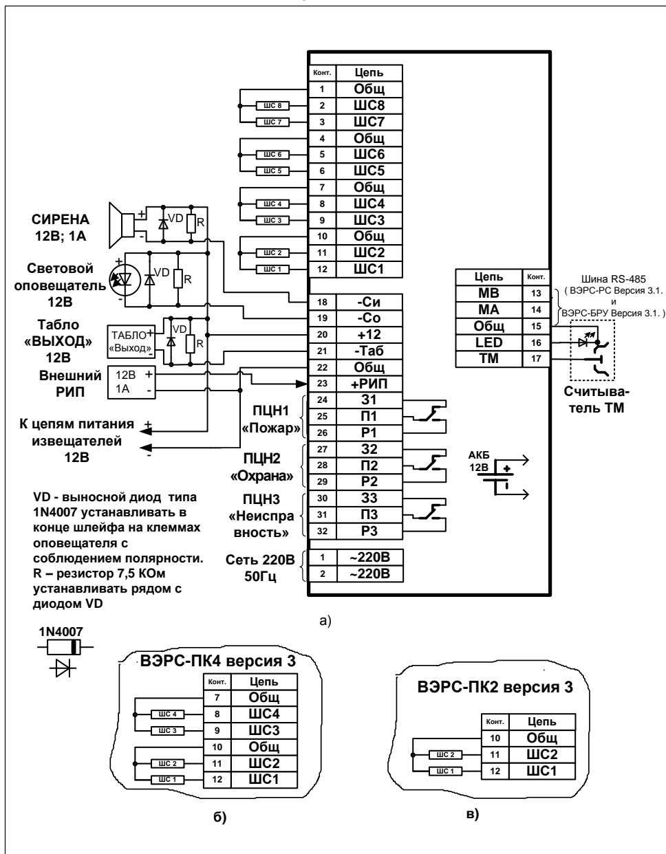
Рисунок.Б1. Схемы внешних соединений приборов ВЭРС-ПК(8,4,2) ТРИО-М.
