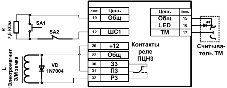
Рисунок Б8. Схема организации Точки доступа.
